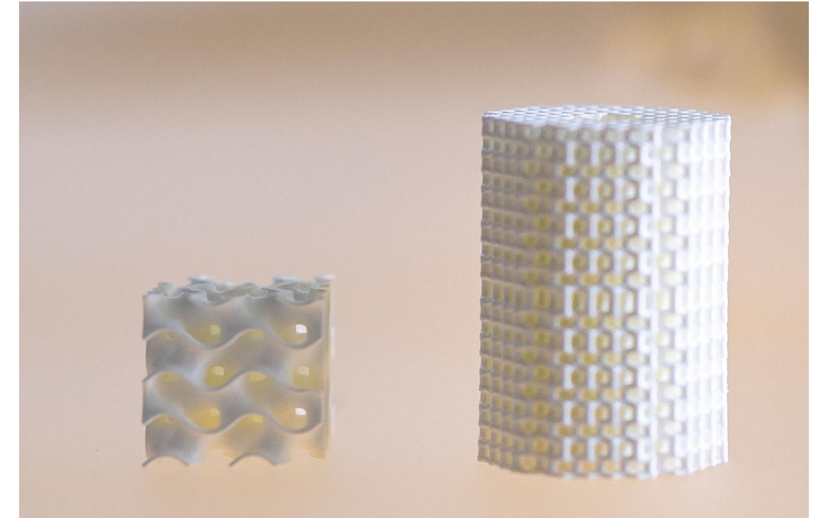
Komplexe Geometrien aus Oxidkeramik gefertigt mittels VPP
